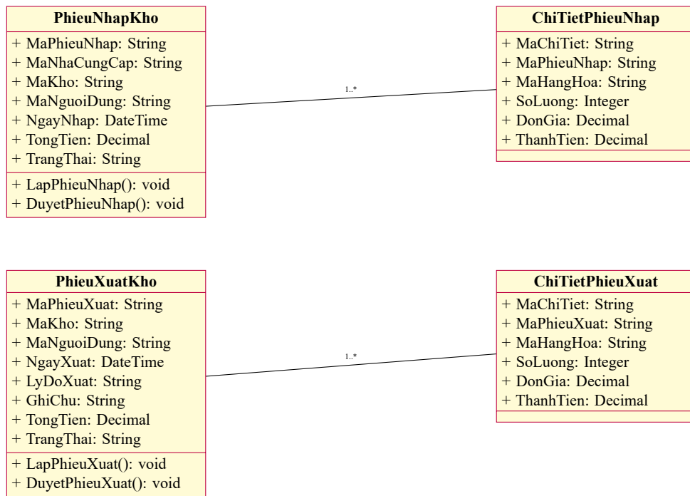
Hình 1: Sơ đồ lớp nghiệp vụ nhập xuất kho
